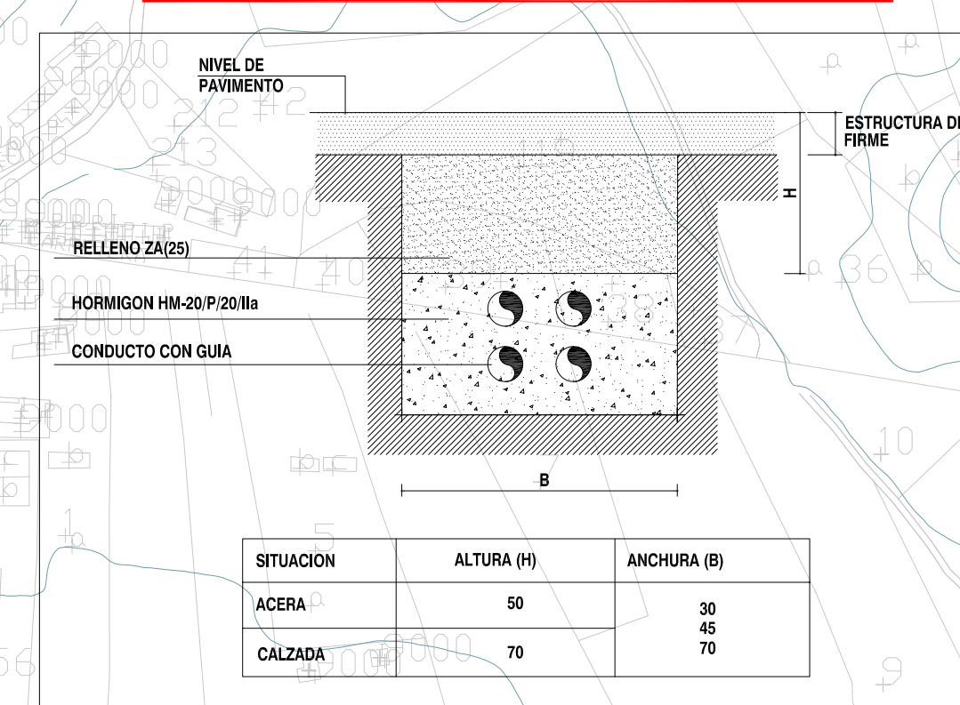
ZANJA PARA ALOJAMIENTO DE LA CONDUCCION SECCION TRANSVERSAL
