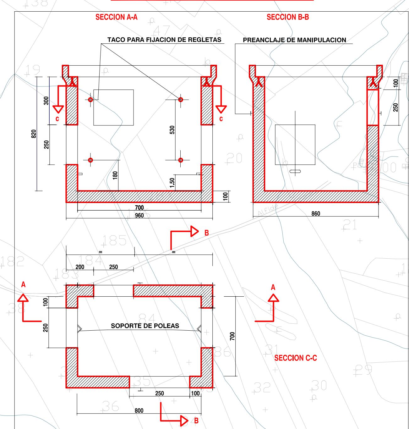
ARQUETA TIPO H.II (PREFABRICADA) DEFINICION GEOMETRICA
