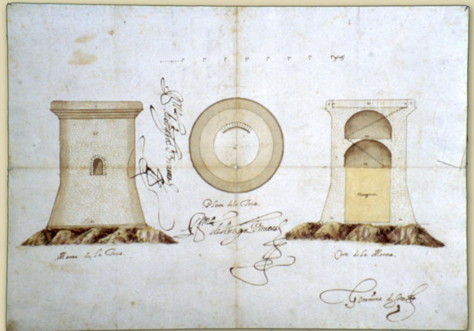
Plano, corte y elevación de una torre que se había de levantar en Cabo Dique y Colindarín. 1625. UMS R.P. y B. 1111-21
