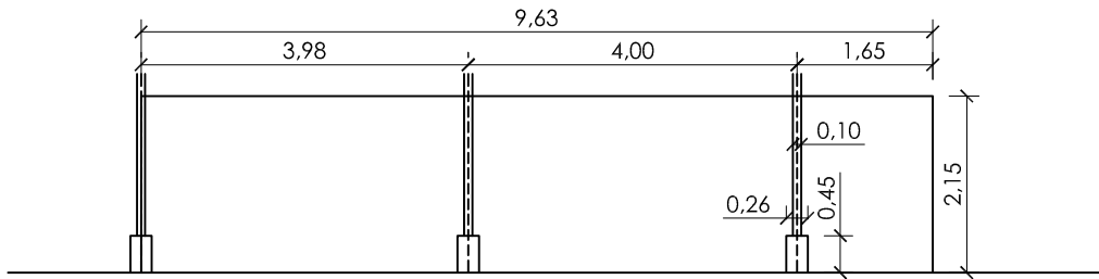
ALZADO DE MEDIANERA PASEO JUNTO AUDITORIO - PASEO PÉRGOLA ESCALA 1:100
