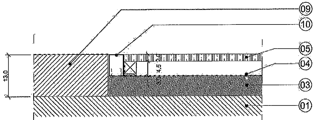
DETALLE ENCUENTRO PERIMETRAL
