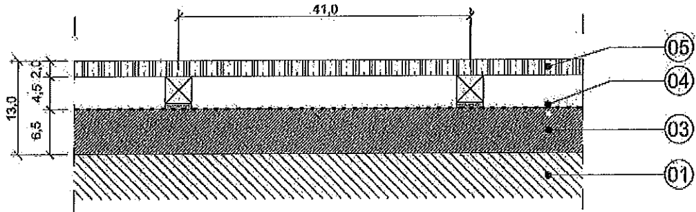
SECCION TIPO PAVIMENTO DEPORTIVO Escala 1/5
