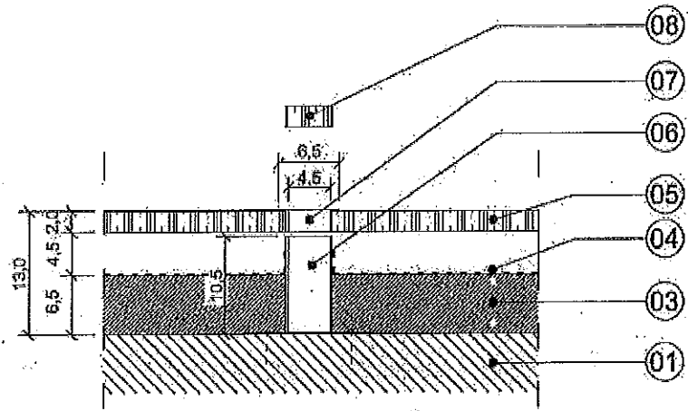
SECCION POR BARANDILLA PERIMETRAL Escala 1/5
