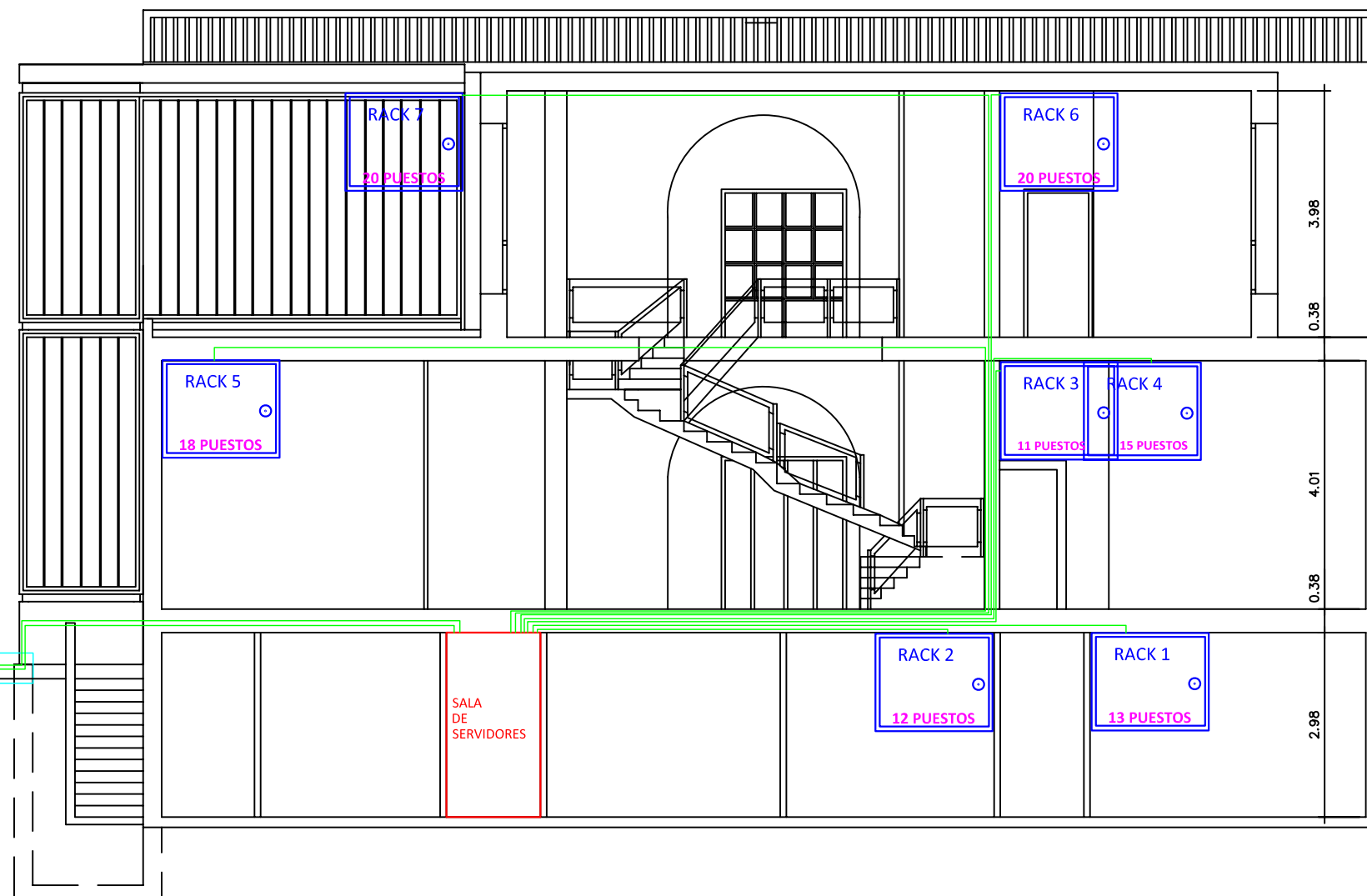
SECCION B-B'
