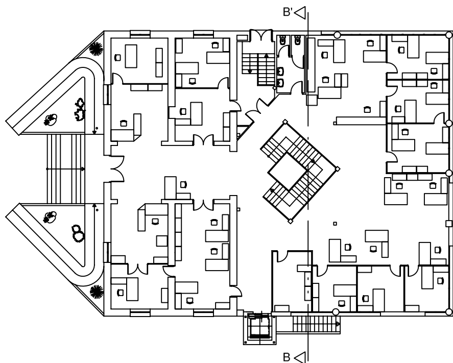
PLANTA DE REFERENCIA: PLANTA BAJA
