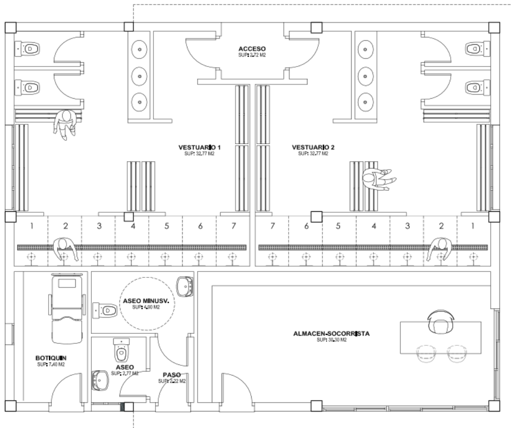
PLANTA ESTADO REFORMADO DISTRIBUCION Y MOBILIARIO ESCALA: 1/50
